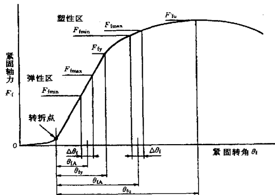
图3 紧固转角与预紧力的关系图
