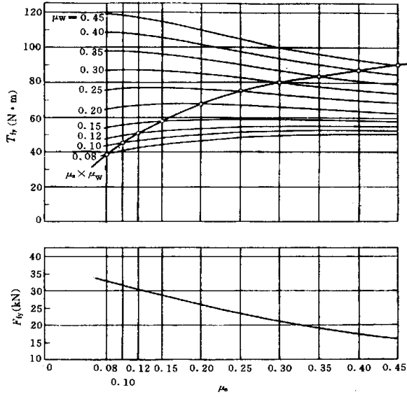
图 B1 \mu_w 和 \mu 与 F_{ty} 和 T_{ty} 的关系图 (M10、8.8)
