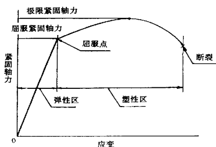
图1 轴力-应变图
