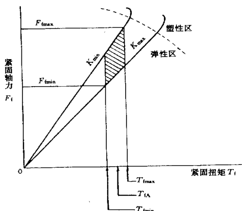
图2 紧固扭矩和预紧力的关系图
