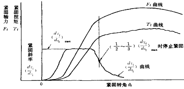
图 4 紧固转角相对应的预紧力及紧固扭矩图
